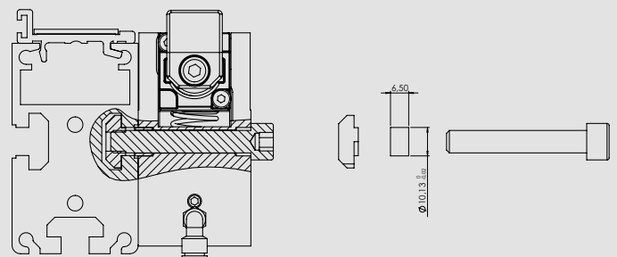
Befestigungssatz B Assembly kit B (44000135)
