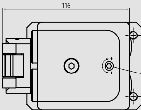
Mit Kippanschlag with tilt stop
