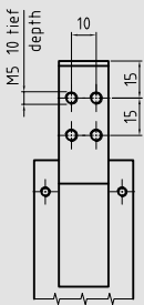
Anschlagplatte mit Gewinde 40 Hub Stop plate with thread 40 stroke
