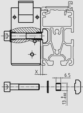
Befestigungssatz B Assembly kit B (44000135)
